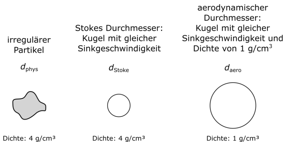
Abbildung 1: Vereinfachter Zusammenhang der unterschiedlichen Durchmesser zur Beschreibung von Partikeln am Beispiel eines Primärpartikels.
